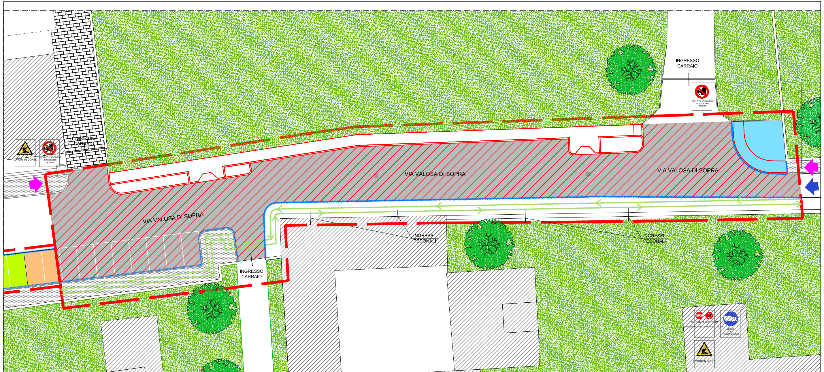
Planimetria fasi di cantiere: Fase 2 - scala 1:500
