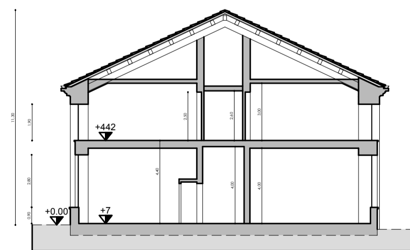
SEZIONE MM'
