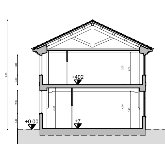
SEZIONE LL'
