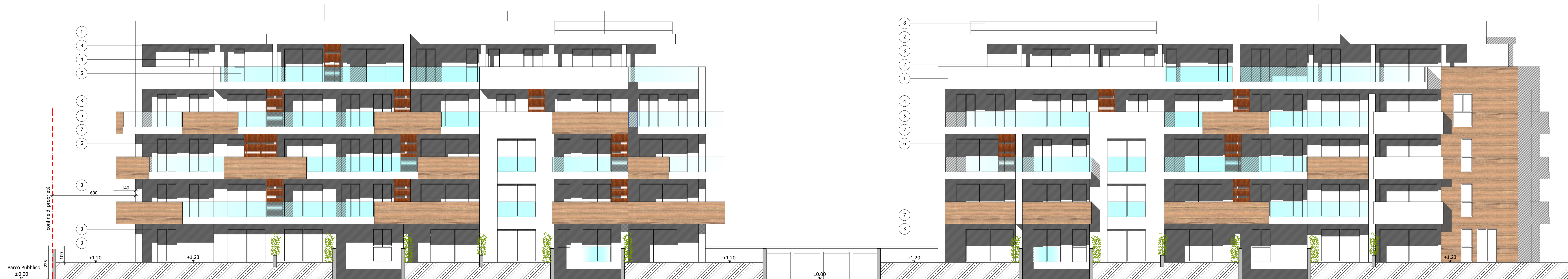
PROSPETTO OVEST - FRONTE PARCO
