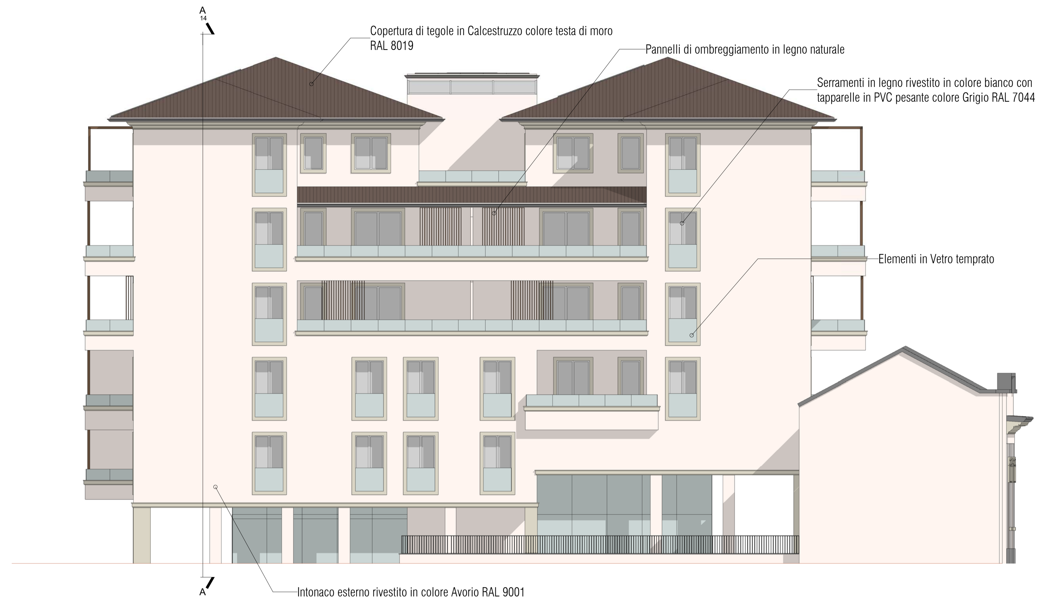
Prospetto Est - Scala 1 : 100
